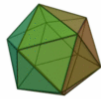
Ikosaeder (Wasser)
