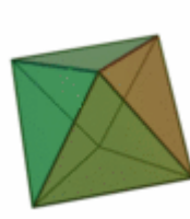
Oktaeder (Luft)
