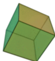
Hexaeder (Erde)
